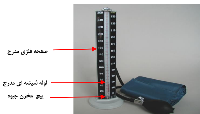
شکل 6:دستگاه فشار سنج جیوه ای(mercury monitor)
